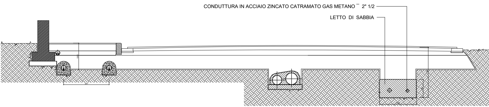
SEZIONE STRADALE SU LINEE DI ADDUZIONE ACQUEDOTTO., GAS 1/50
