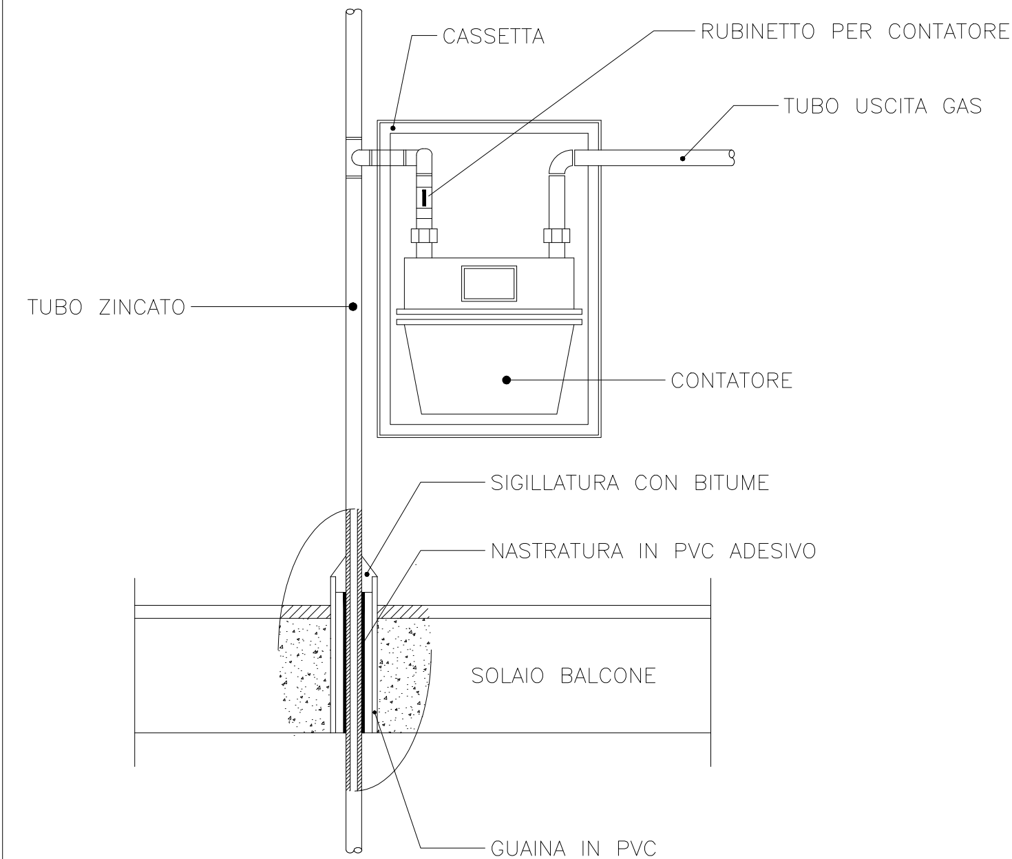
Disegno / schema di un contatore del gas
