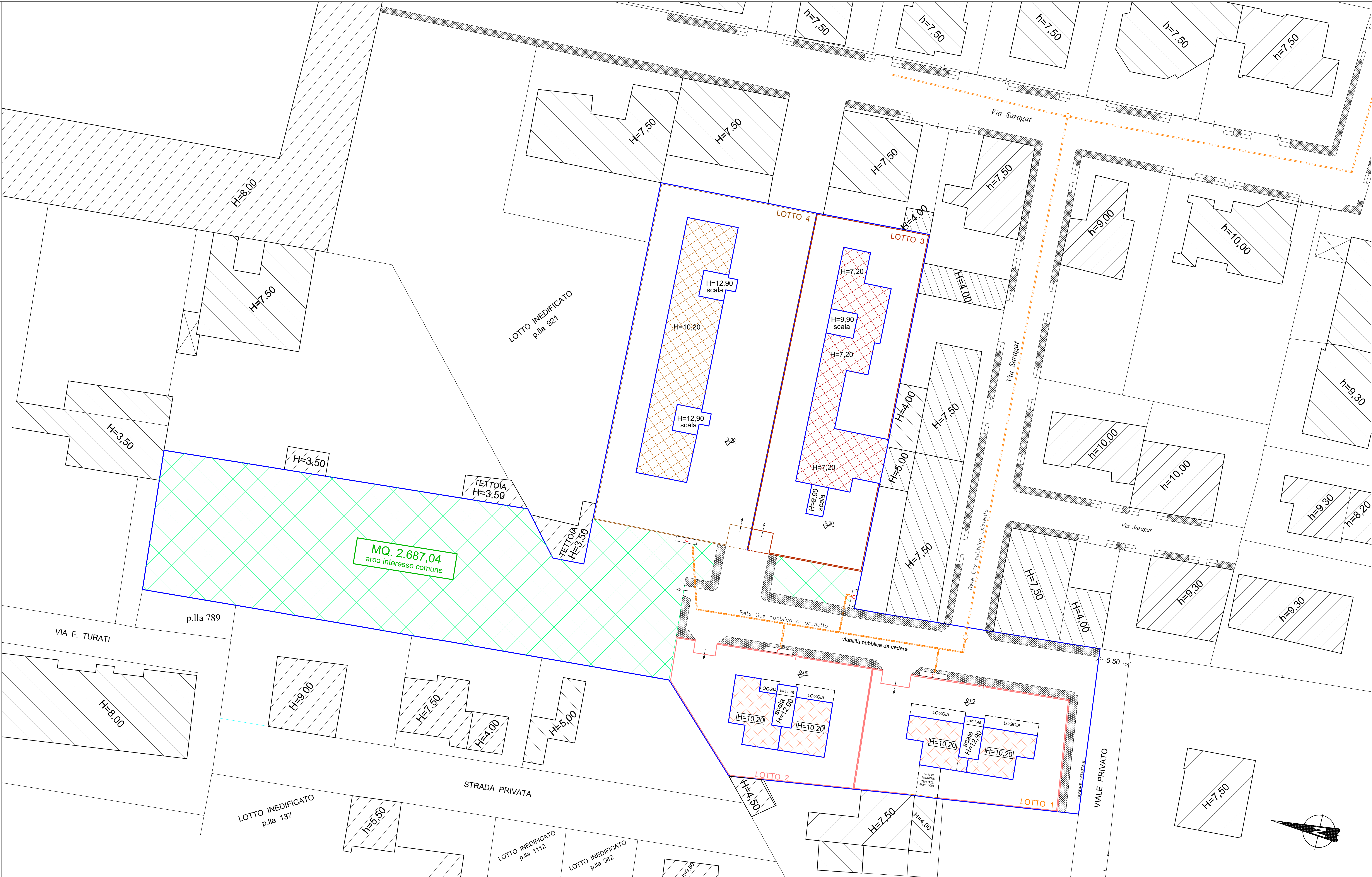
PLANIMETRIA GENERALE IMPIANTO ADDUZIONE GAS SCALA 1- 300
