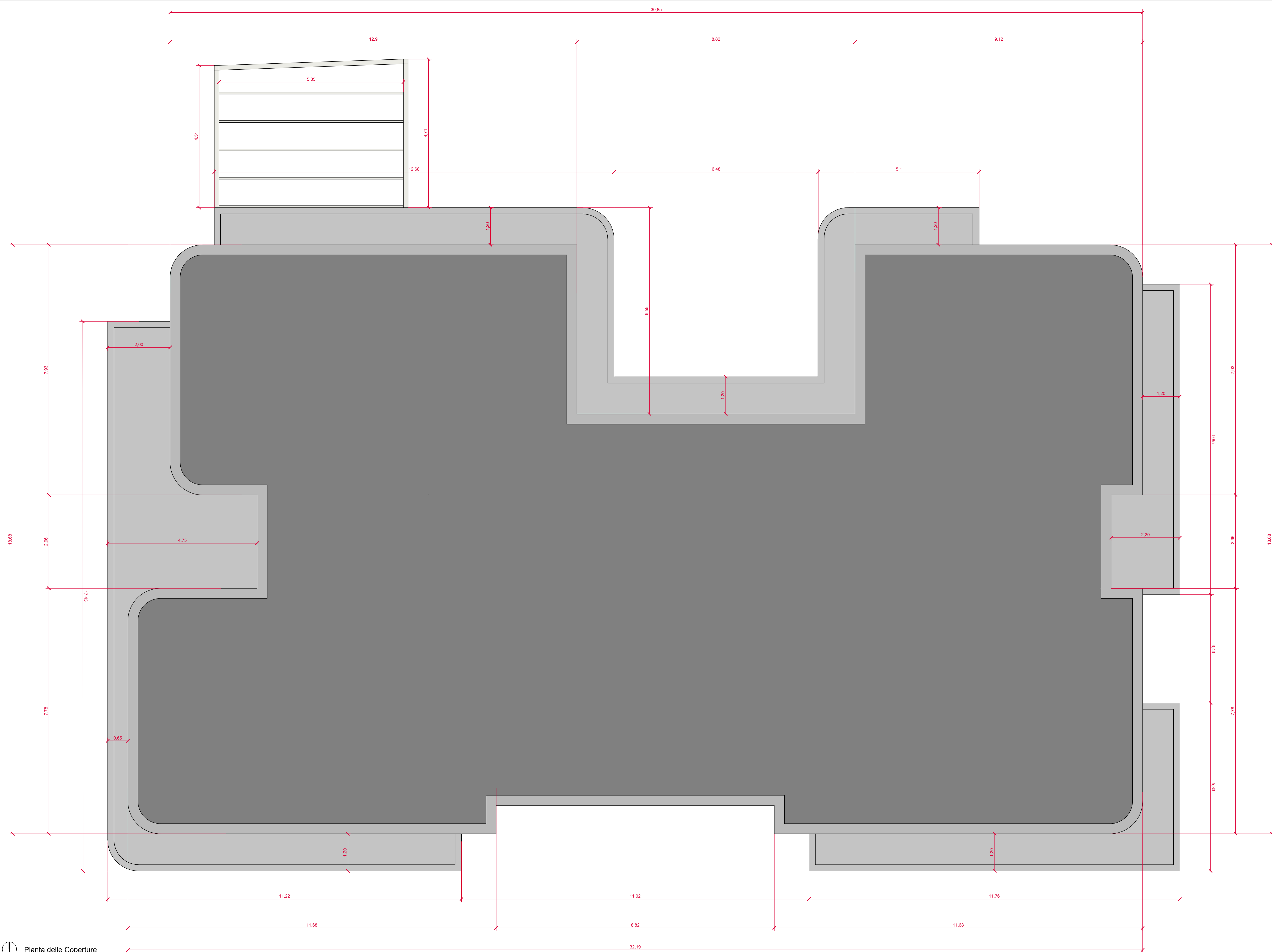
⊕ Pianta delle Coperture
