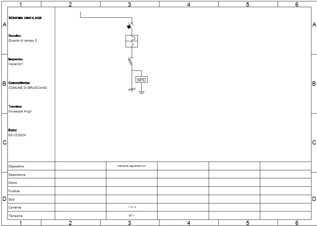
Fig. 7: Schema unifilare quadro "Quadro di campo 2"
