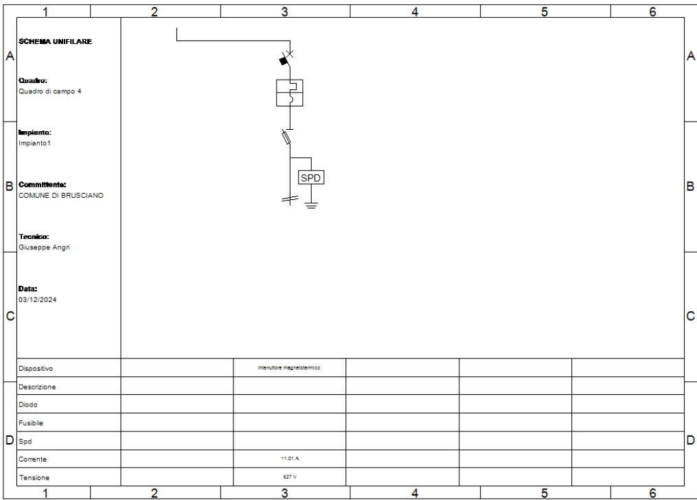
Fig. 9: Schema unifilare quadro "Quadro di campo 4"
