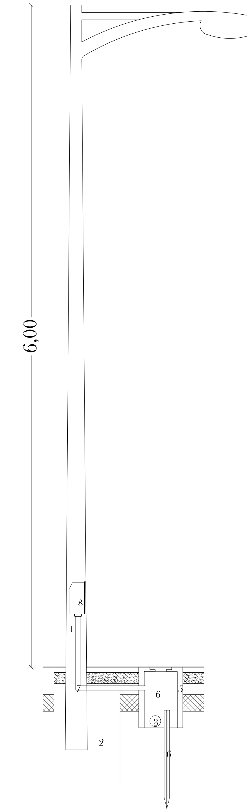
SEZIONE IMPIANTO ILLUMINAZIONE PUBBLICA CON UNA SOLA ARMATURA STRADALE 1:20
