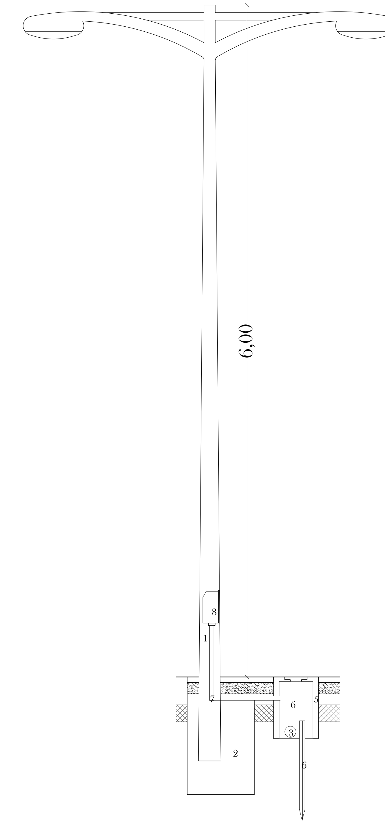
SEZIONE IMPIANTO ILLUMINAZIONE PUBBLICA CON DOPPIA ARMATURA STRADALE 1:20
