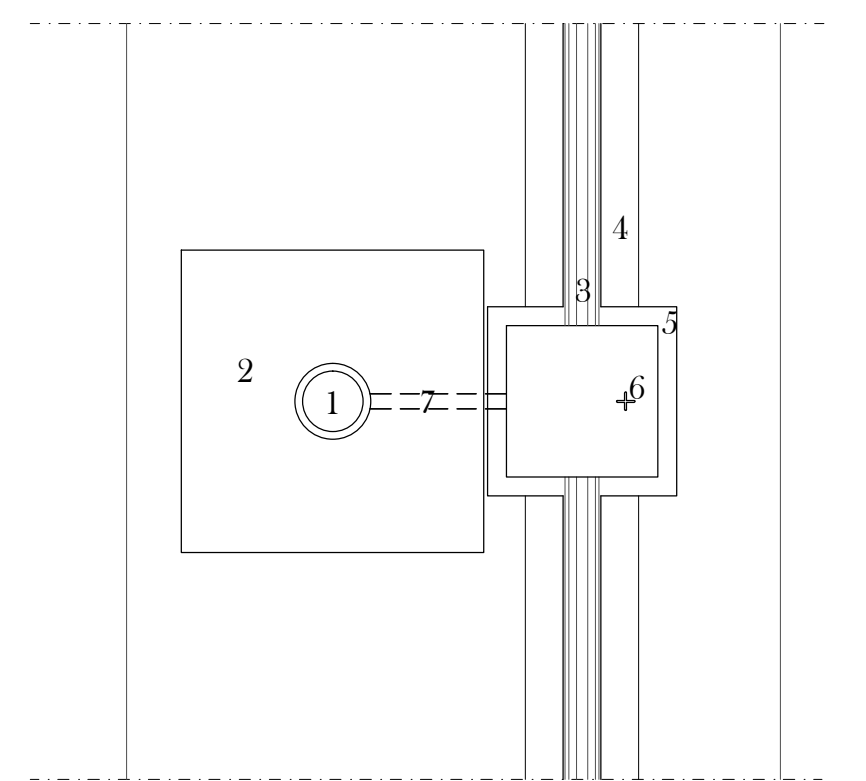
PIANTA IMPIANTO ILLUMINAZIONE PUBBLICA 1:20
