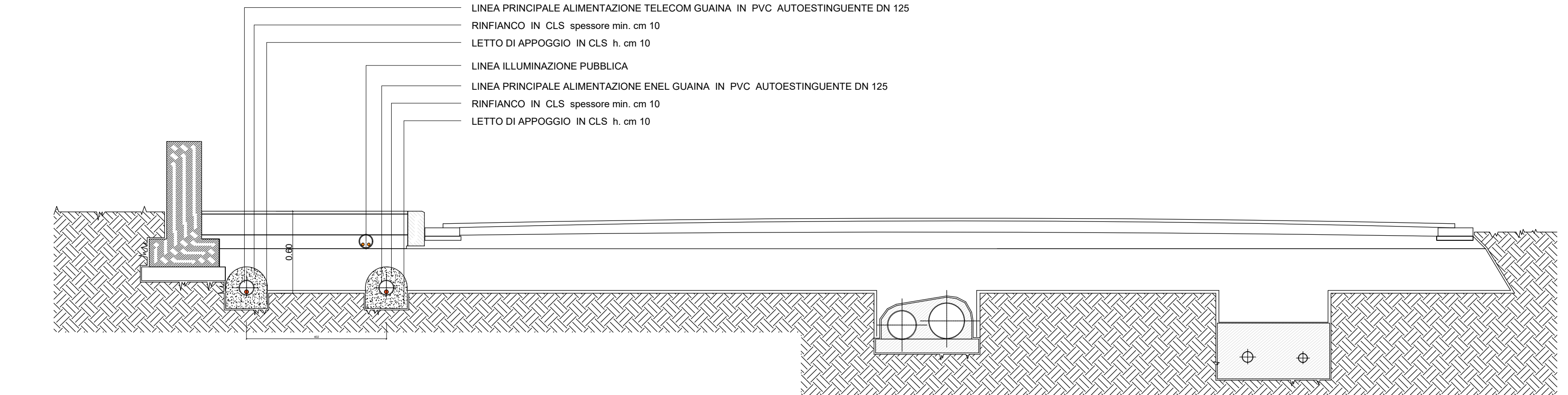
SEZIONE STRADALE SU LINEE DI ADDUZIONE , ELETTRICA, 1/25
