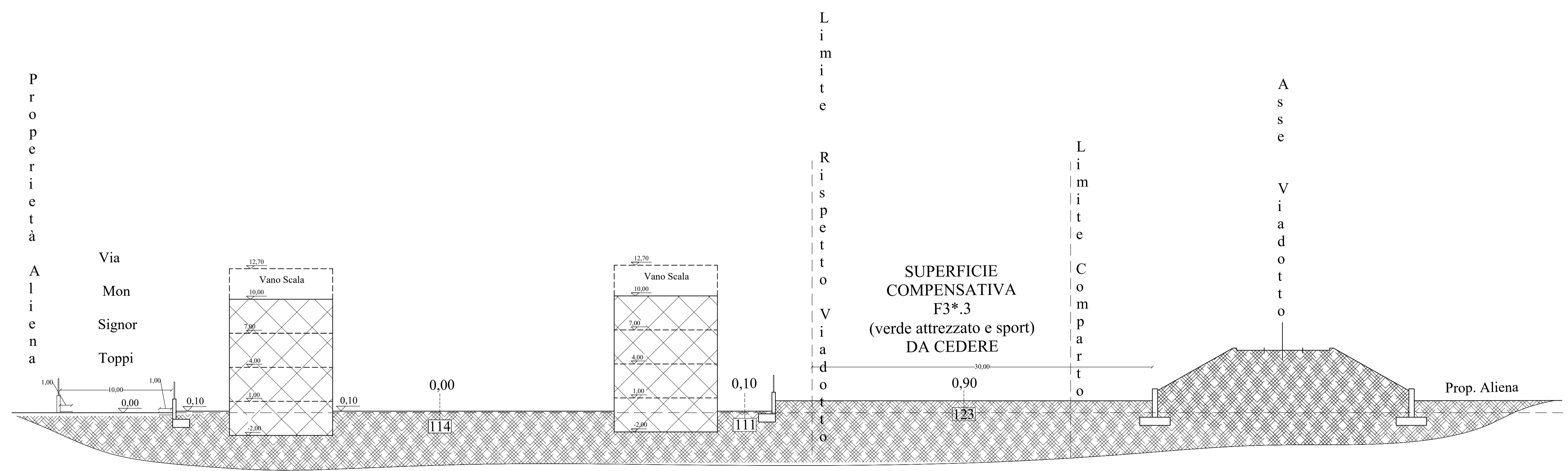
PROFILO B-B SCALA 1-200
